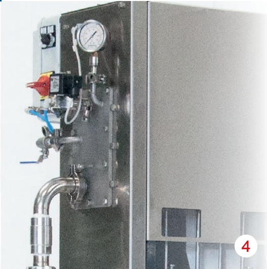
Bildlegende: 1) Karbonisatorpumpe, 2) Pneumatisch betätigte Füllinheit, 3) Trockenlaufschutz, 4) Druckregleinheit für CO 2 & Anschluss für karbonisierte Flüssigkeiten, 5) Kronenkorkverschleißer
